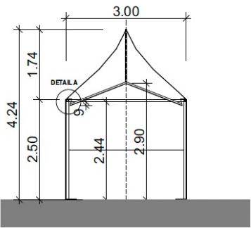
QUERSCHNITT PAGODENZELT 3X3 METER
