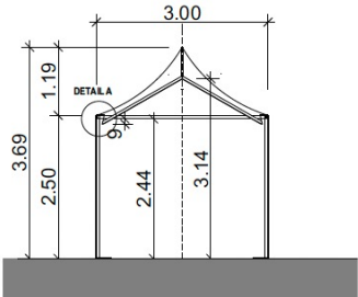
QUERSCHNITT PAGODENZELT 3X5 METER CITY
