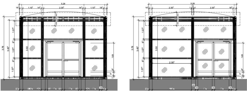
FASSADEN MANHATTAN CUBE 5X10 METER 5 METER SEITE
