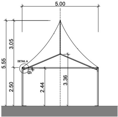
QUERSCHNITT PAGODENZELT 5X5 METER
