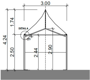
QUERSCHNITT PAGODENZELT 3X3 METER
